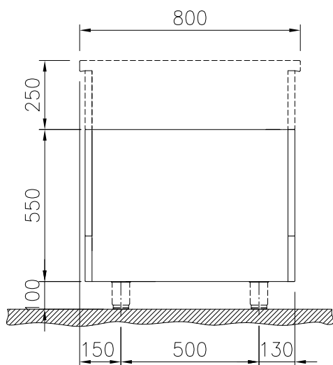
Zij aanzicht
